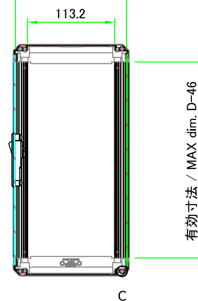
有効寸法 / MAX dim. 144
